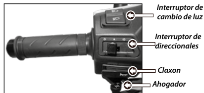
Imagen 4. Mando izquierdo.
