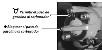
Imagen 11. Válvula de combustible.
