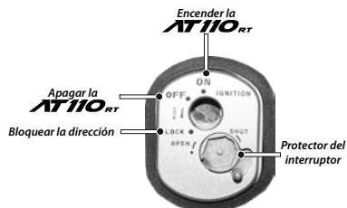
Imagen 9. Interruptor de encendido y bloqueo.
