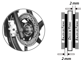
Imagen 21. Desgaste del freno delantero.
