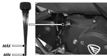
Imagen 16. Bayoneta del cárter.
