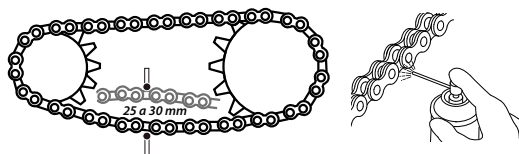
Imagen 24. Holgura de la cadena.
